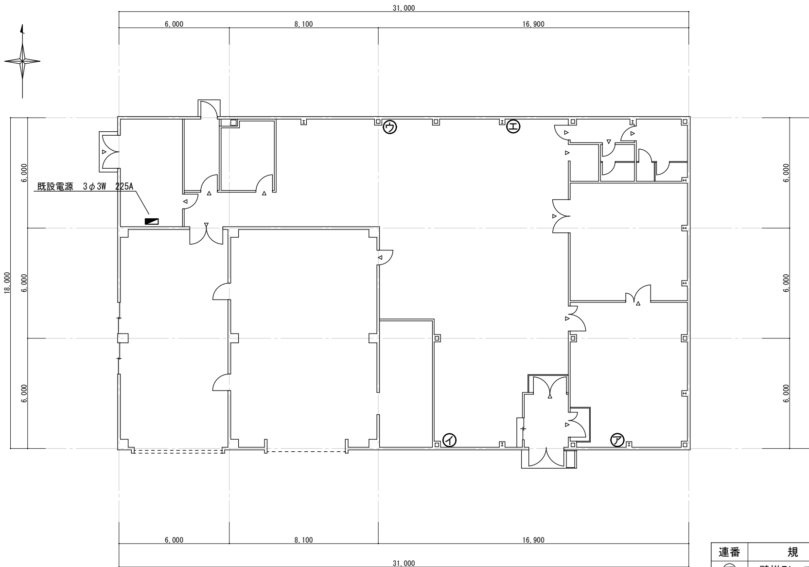
640号建物平面図 S=1/200
