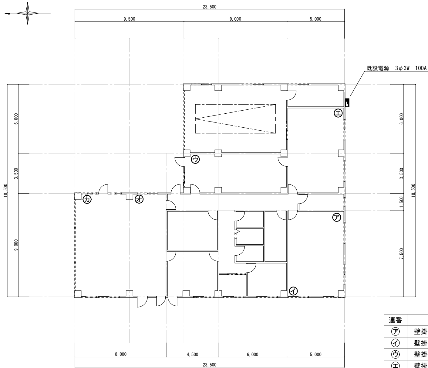
39号建物平面図 S=1/200
