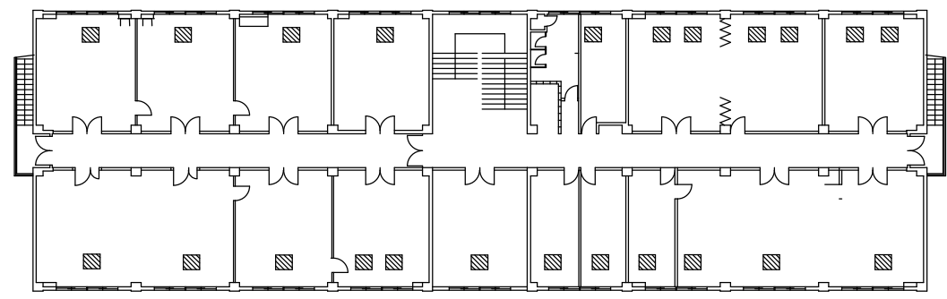
566号建物2F平面図 S=1/300
