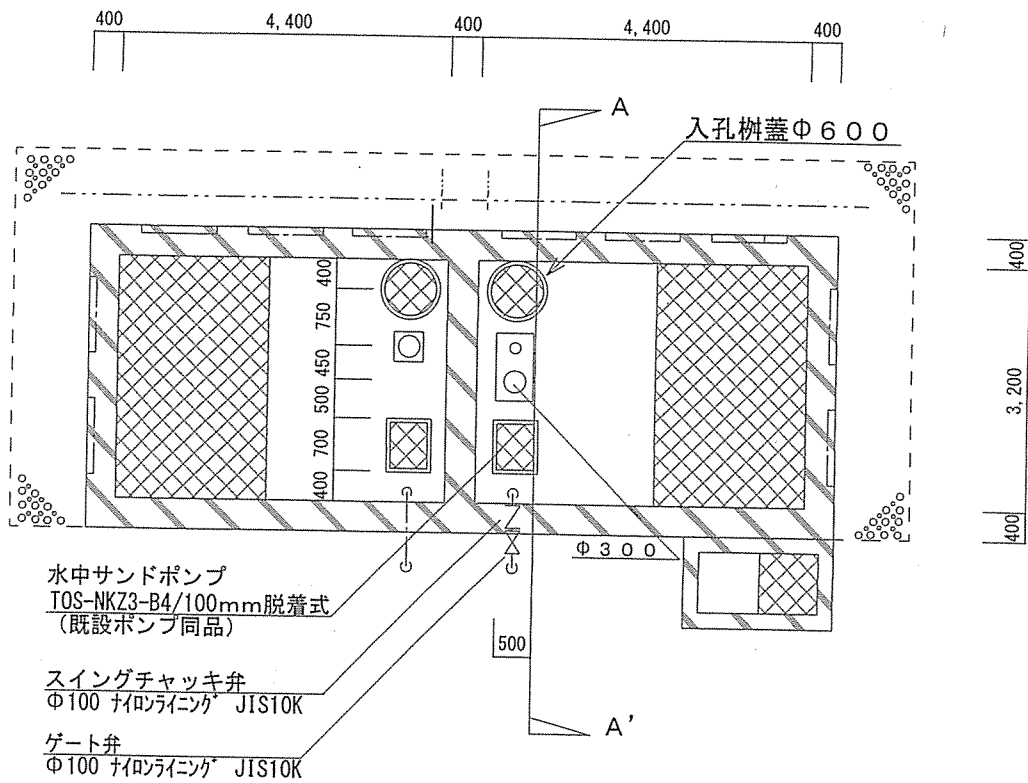
平面図 S=1/100
