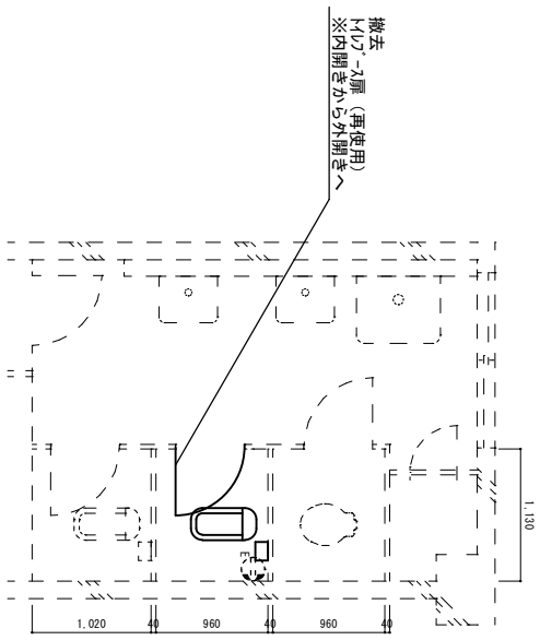
本部隊舎1階女子便所改修前平面図 S=1:50
