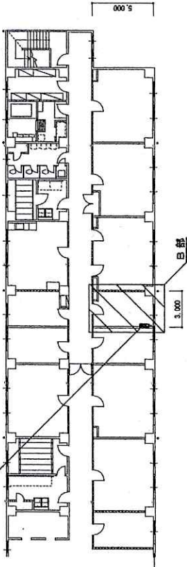
生活隊舎7階東側平面図 S=1:300
