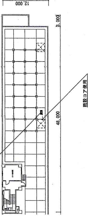
生活隊舎屋上平面図 S=1:300
