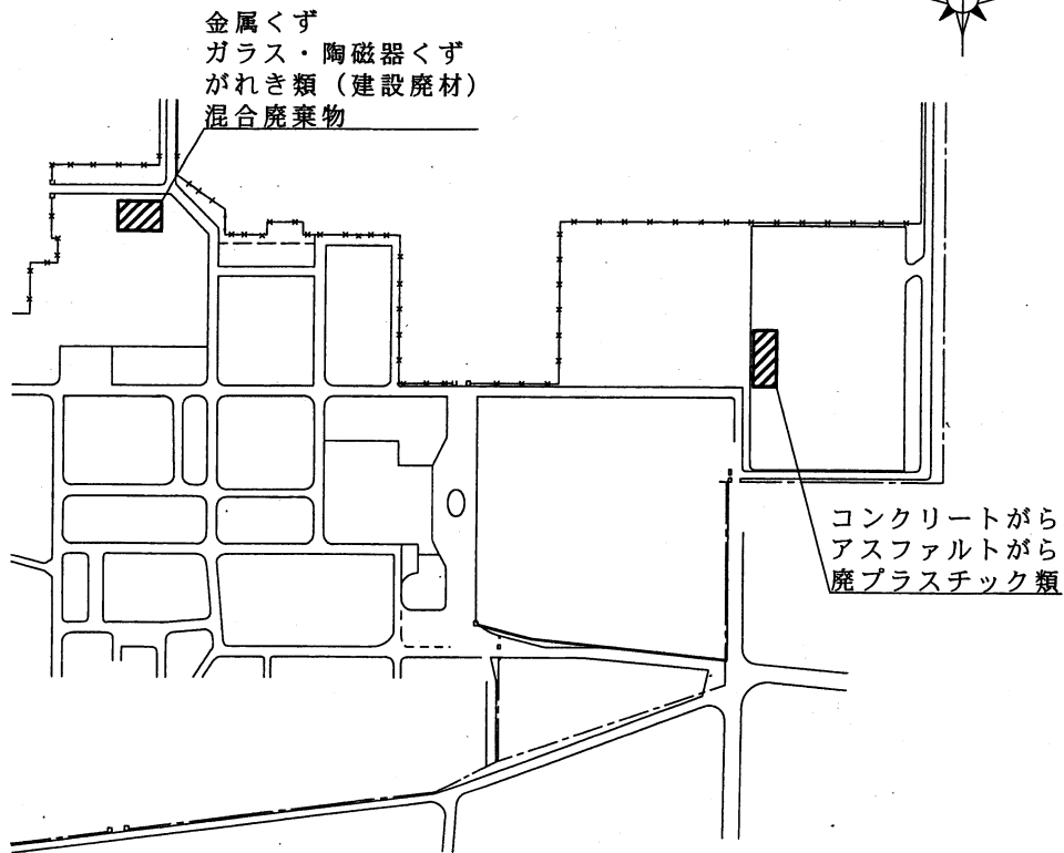
配置図 S=1:X
