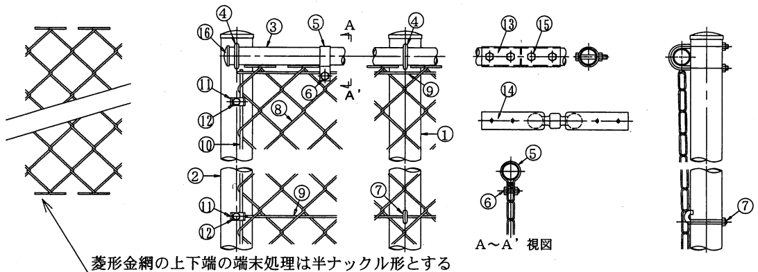
外柵フェンス詳細図 S=1/X
