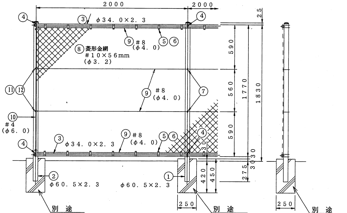
外柵フェンス姿図 S=1/X
