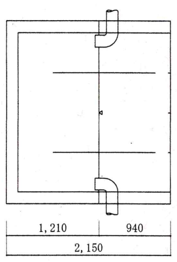
油分離槽 1/50
