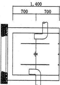
No.10油分離槽 S=1:70
