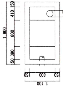
No.10油分離槽 S=1:70
