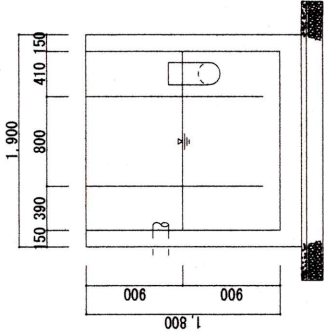
No.12油分離槽 S=1:70
