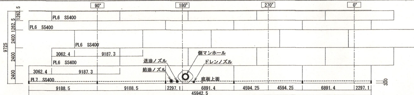
側板配列図 S=1:250
