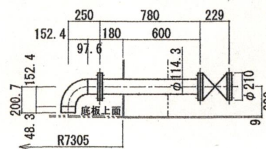
100A ドレンノズル詳細図 S=1:40
