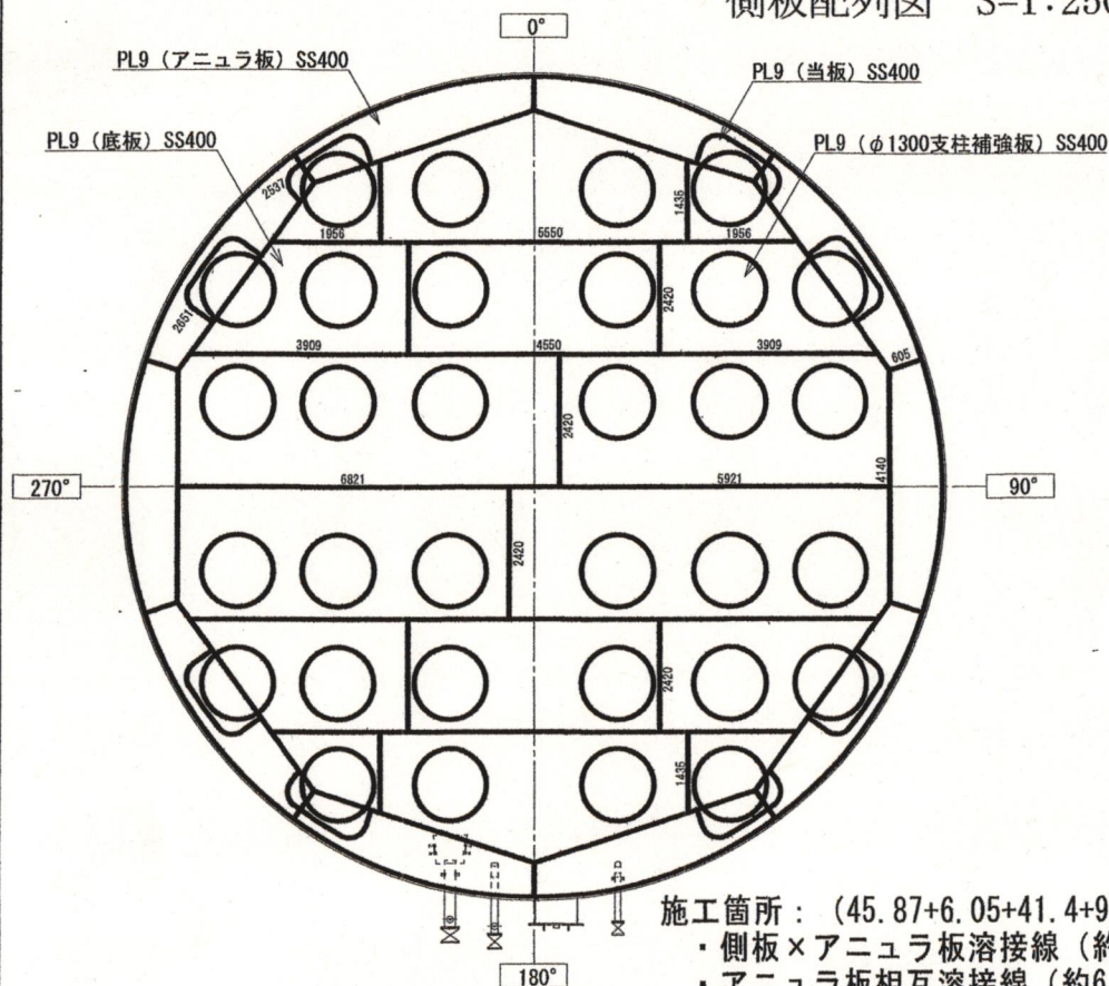
タンク底板詳細図 S=1:150
