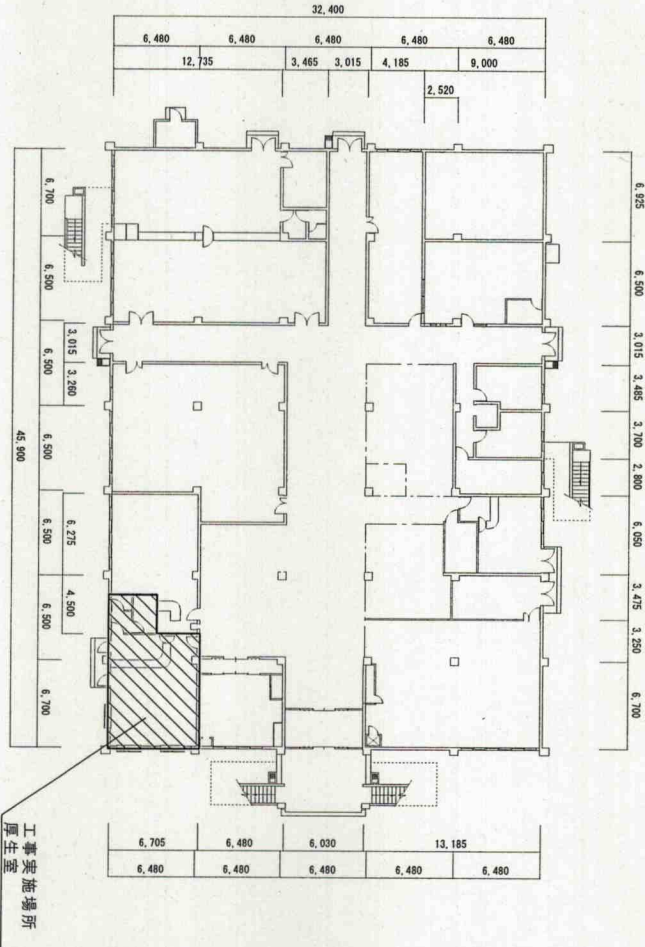
216号 1階平面図 1:400
