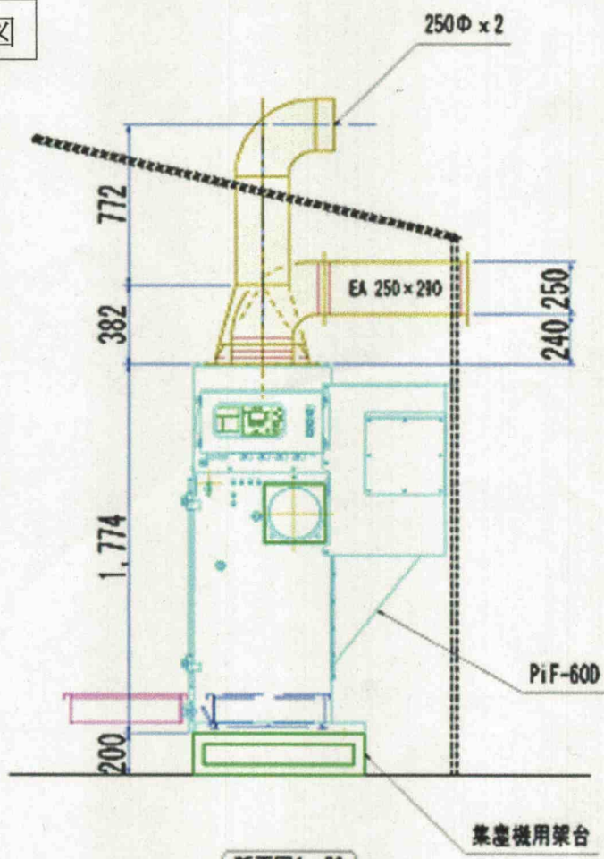
断面図 1 : 30
