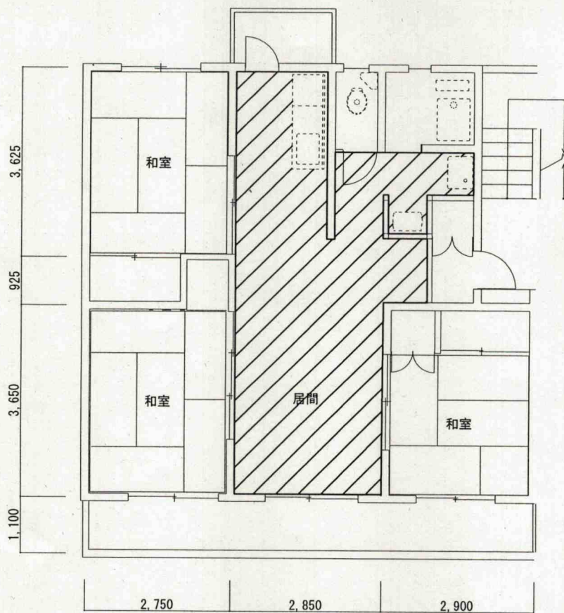
上峰宿舎B棟標準平面図 1 : 1 0 0
