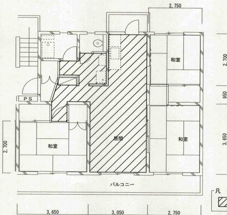
目達原宿舎1号棟標準平面図 1 : 1 0 0
