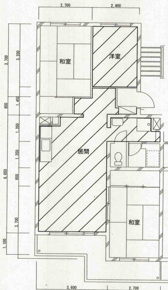
上峰宿舎C棟標準平面図 1 : 100
