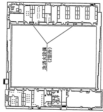
240号格納庫平面図 1/700
