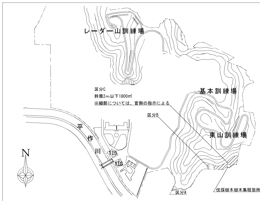
配置図 S=1/8000
