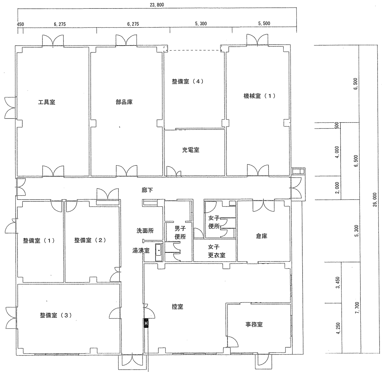
110号館平面図（事務所）S=1/200
