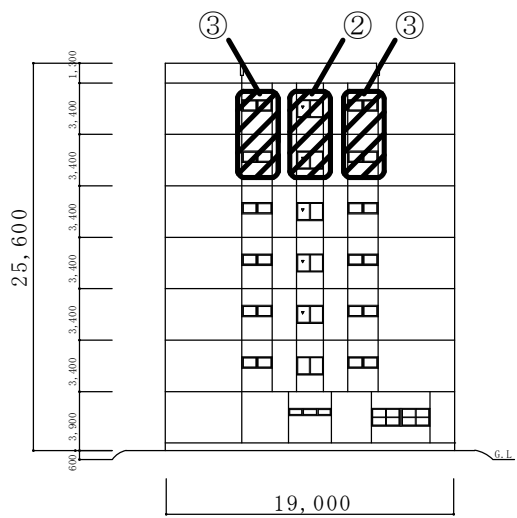
100号館西側立面図 1:500
