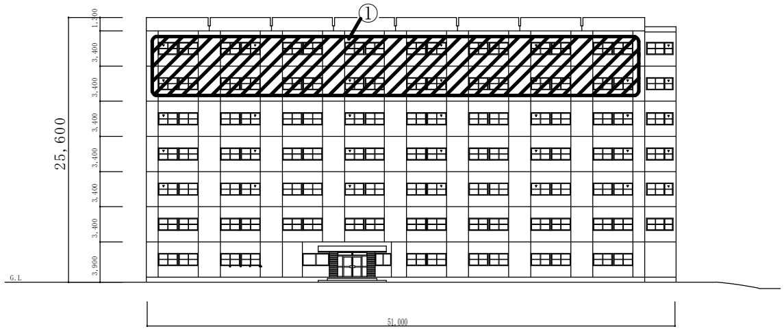
100号館南側立面図 1:500
