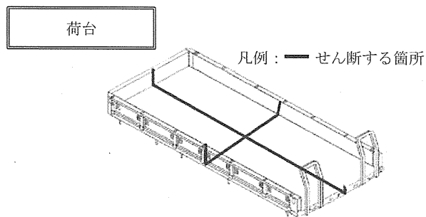
図3-大型トラック外装部品及びフレームの解体・破碎図
