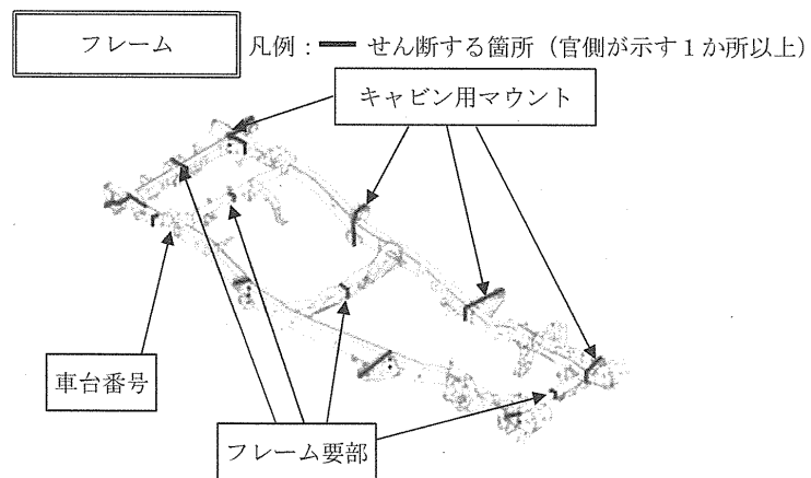
図1-小型トラック外装部品及びフレームの解体・破碎図
