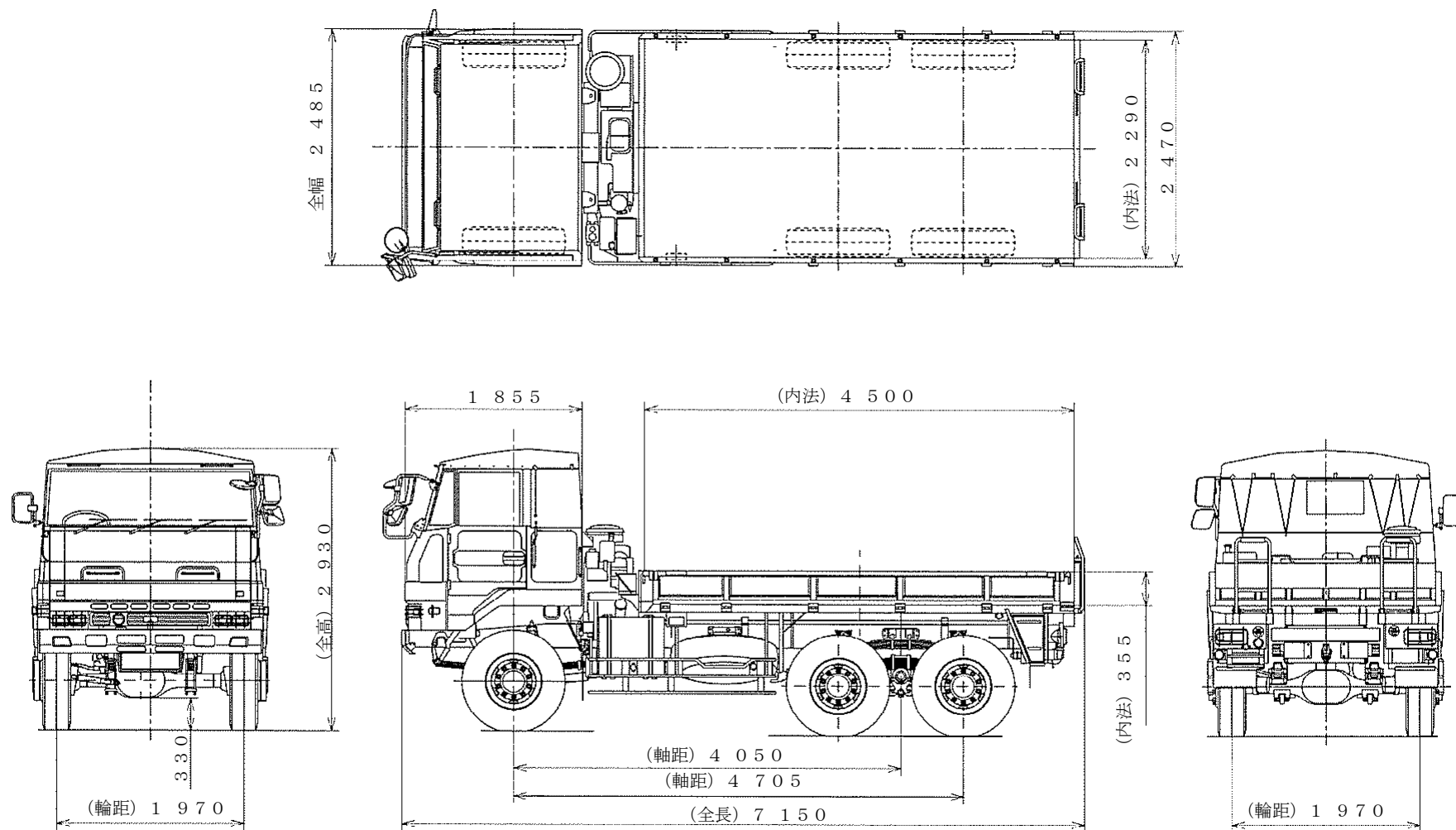
図1-3 \frac{1}{2} tトラック（搭載用）
