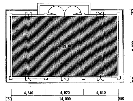
172号倉庫平面図 1:100
