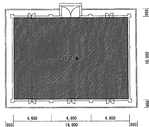
173号倉庫平面図 1:100
