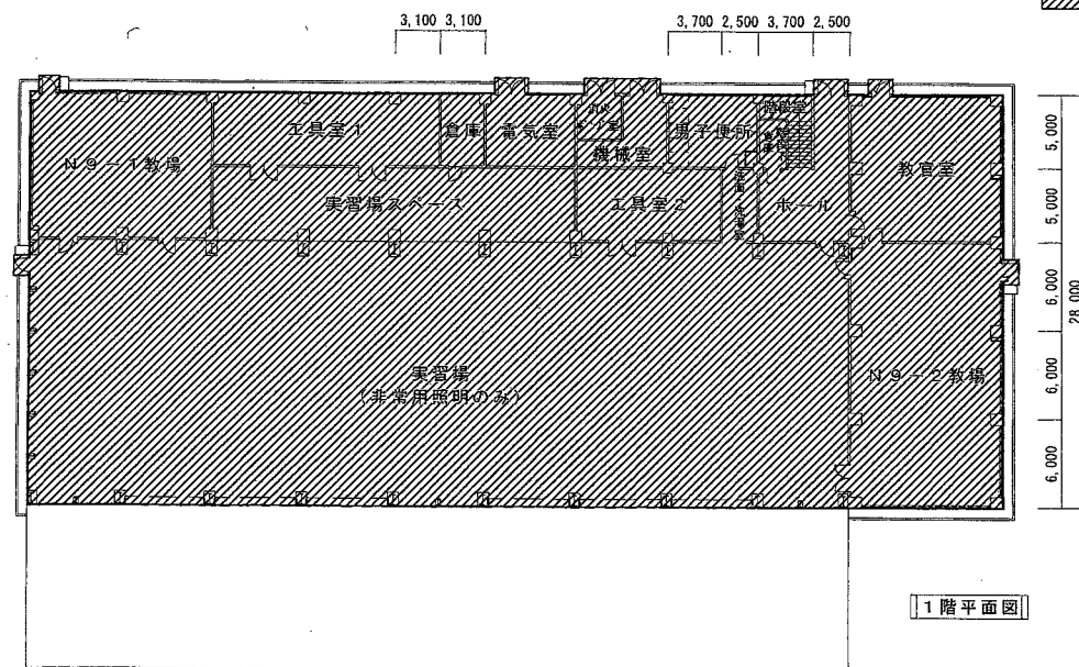
171号実習場平面図 1:400
