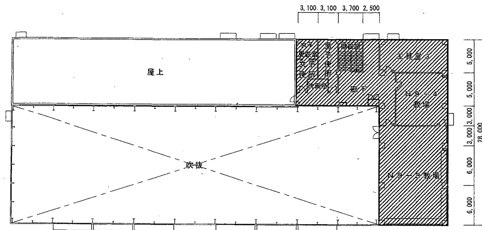
2階平面図
