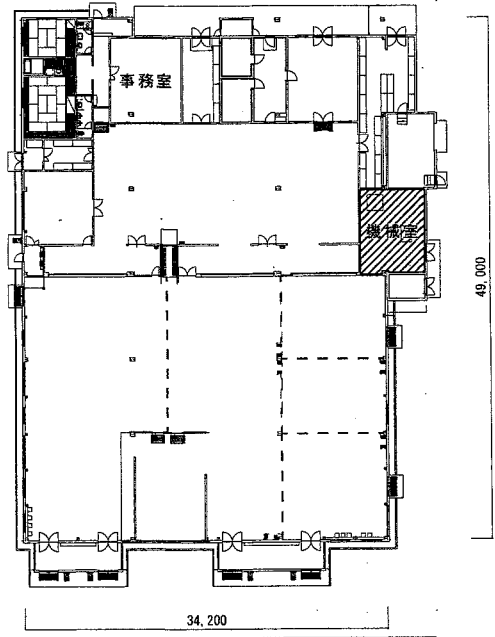
16号食堂厨房平面図 S=1:500
