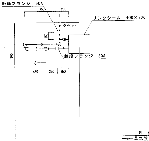
16号食堂厨房地下ピット内蒸気管平面図 S=1:30
