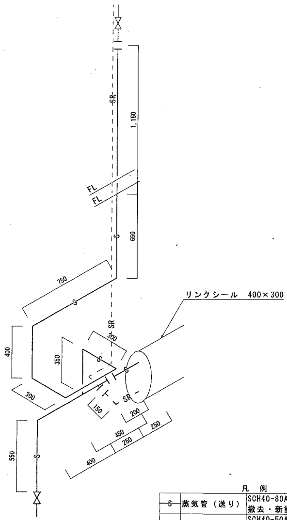
16号食堂厨房地下ピット内蒸気管系統図 S=1:20
