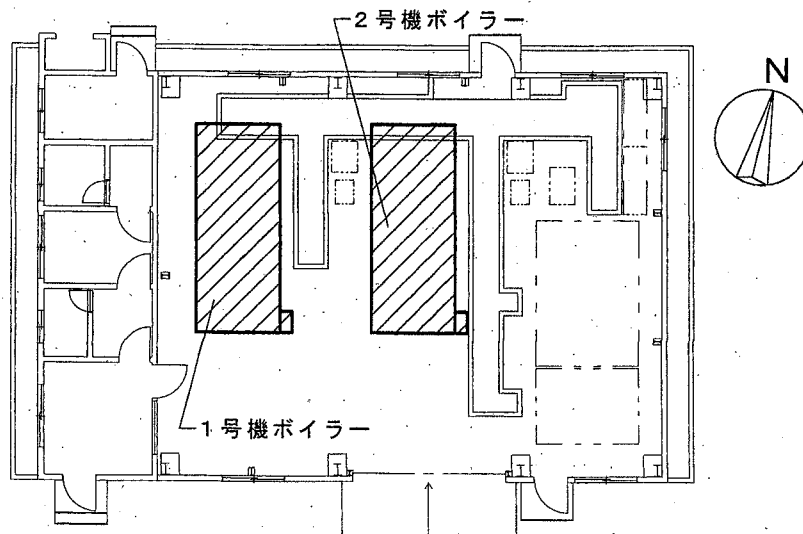
ボイラー室平面図 S=1:X
