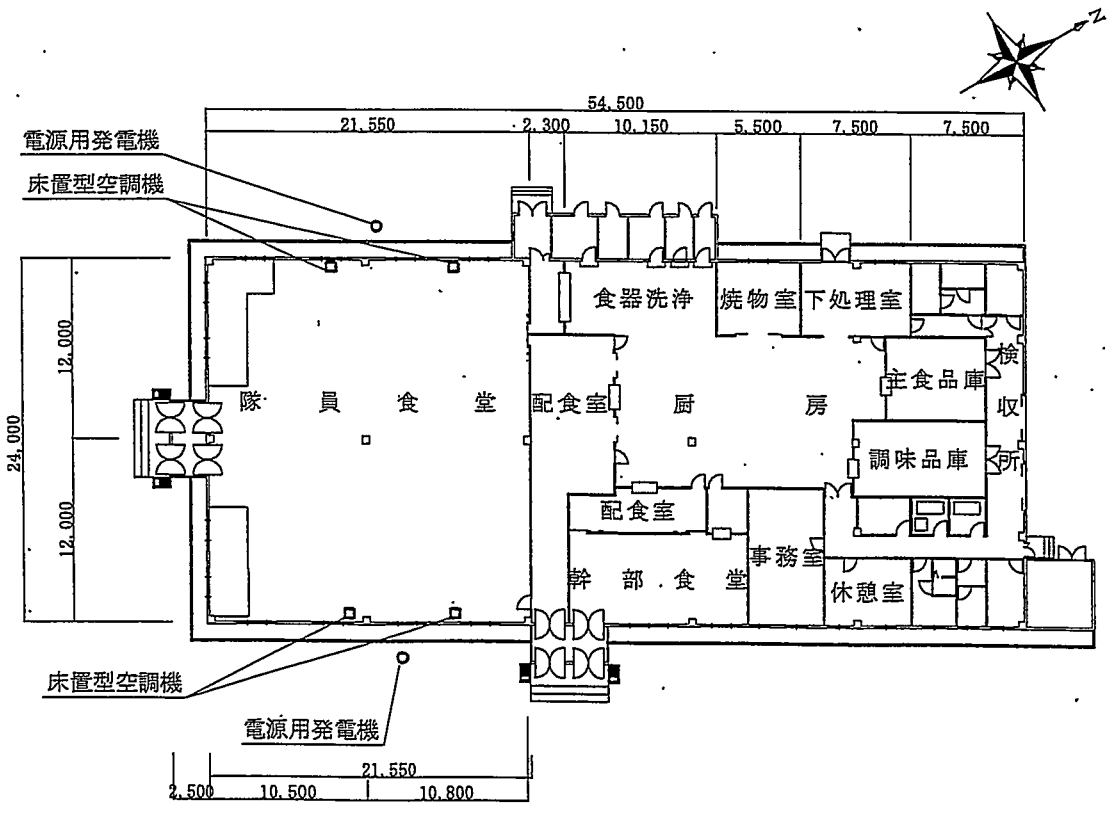
#12隊員食堂平面図 S=1:200
