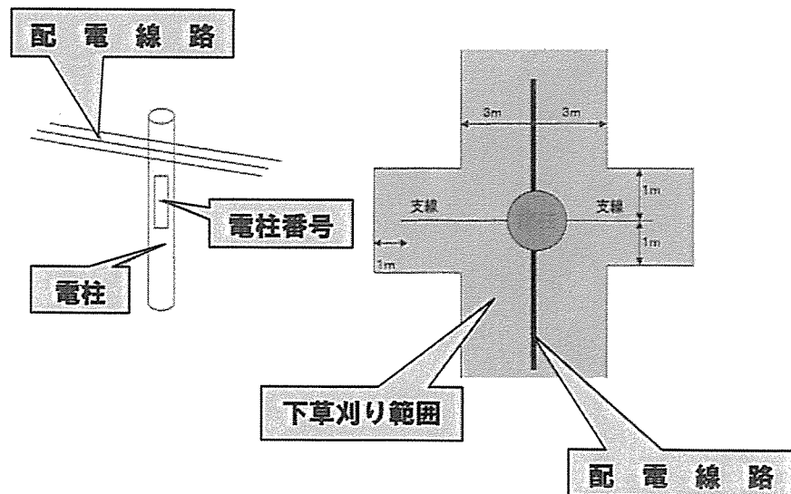
下草刈り範囲（標準図）
