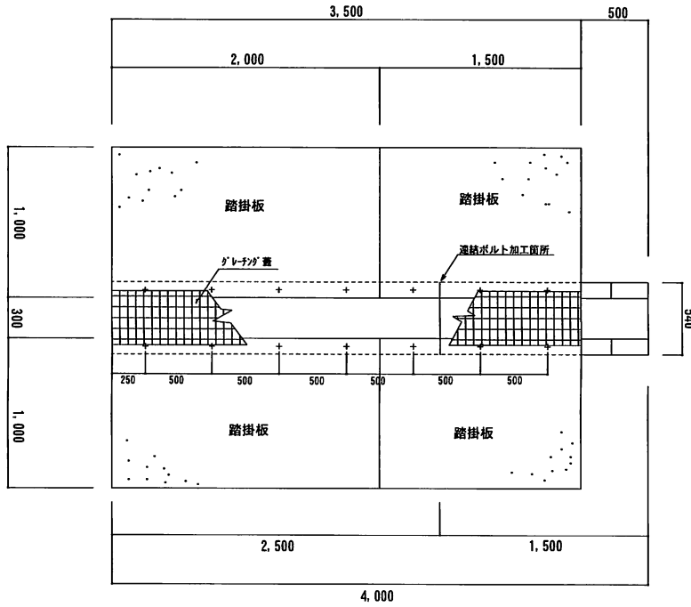
平面図 1 : 50
