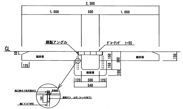
断面図 1 : 30
