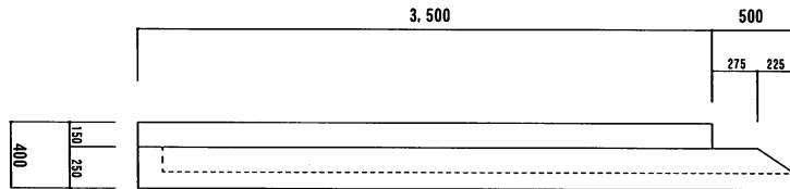
側面図 1 : 50
