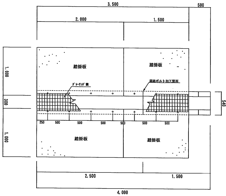
平面図 1 : 50
