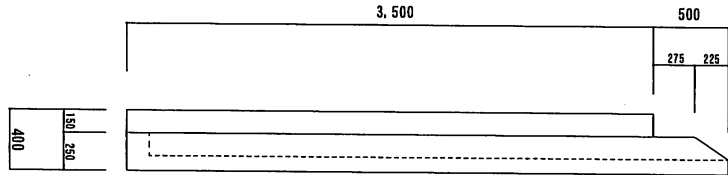
側面図 1 : 50
