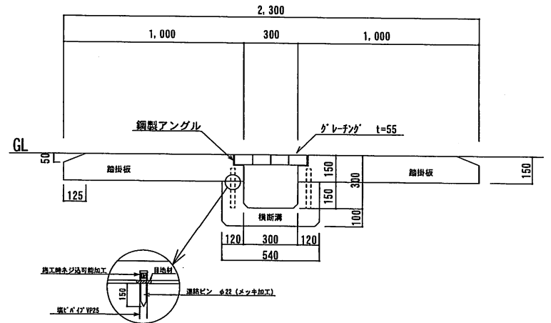
断面図 1 : 30
