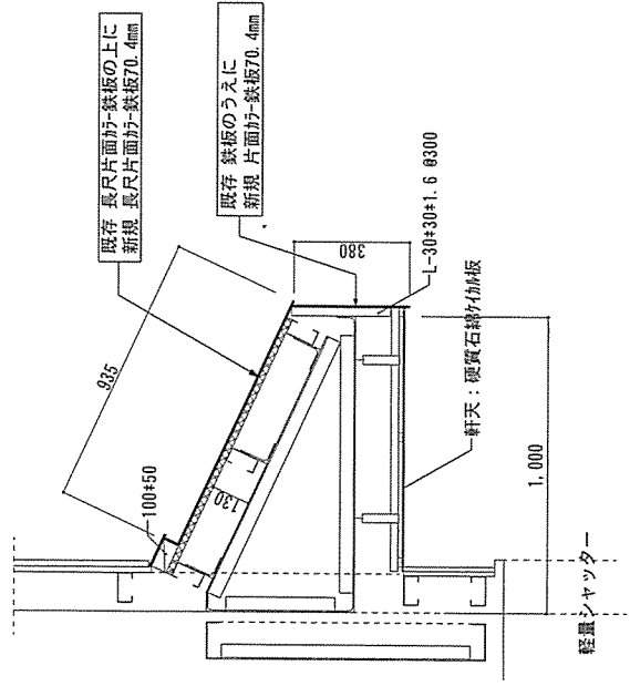
シャッター上部庇部詳細図 S=1:20
