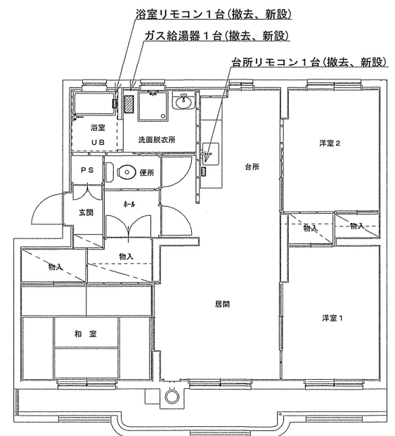
1号棟109号室平面図 S=1:100
