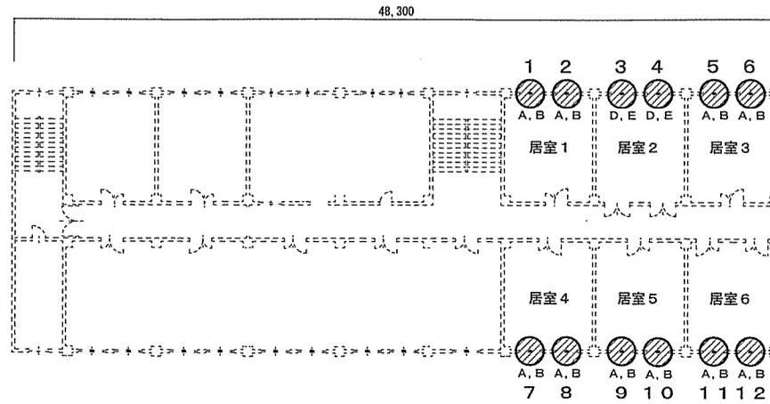
# 5 2 隊舎 ( 3 F ) 平面図 S=1:300
