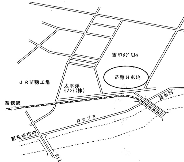
案内図 S=1:12,500
