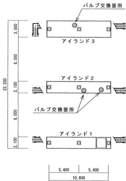
燃料スタンド平面図 S=1:300
