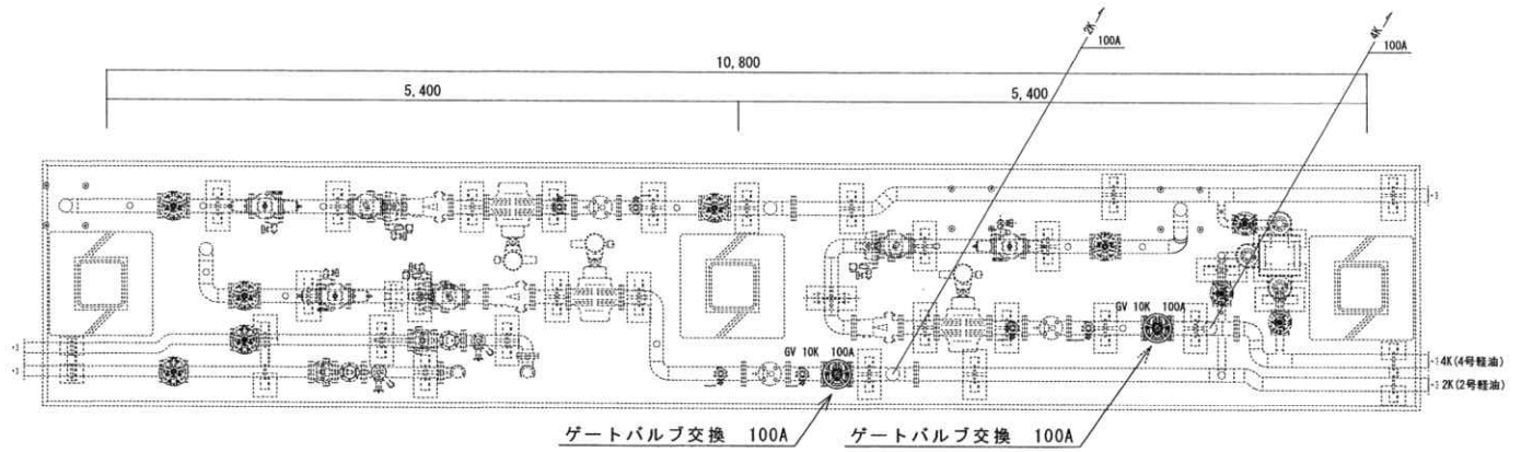
アイランド2 平面図 S=1:50
