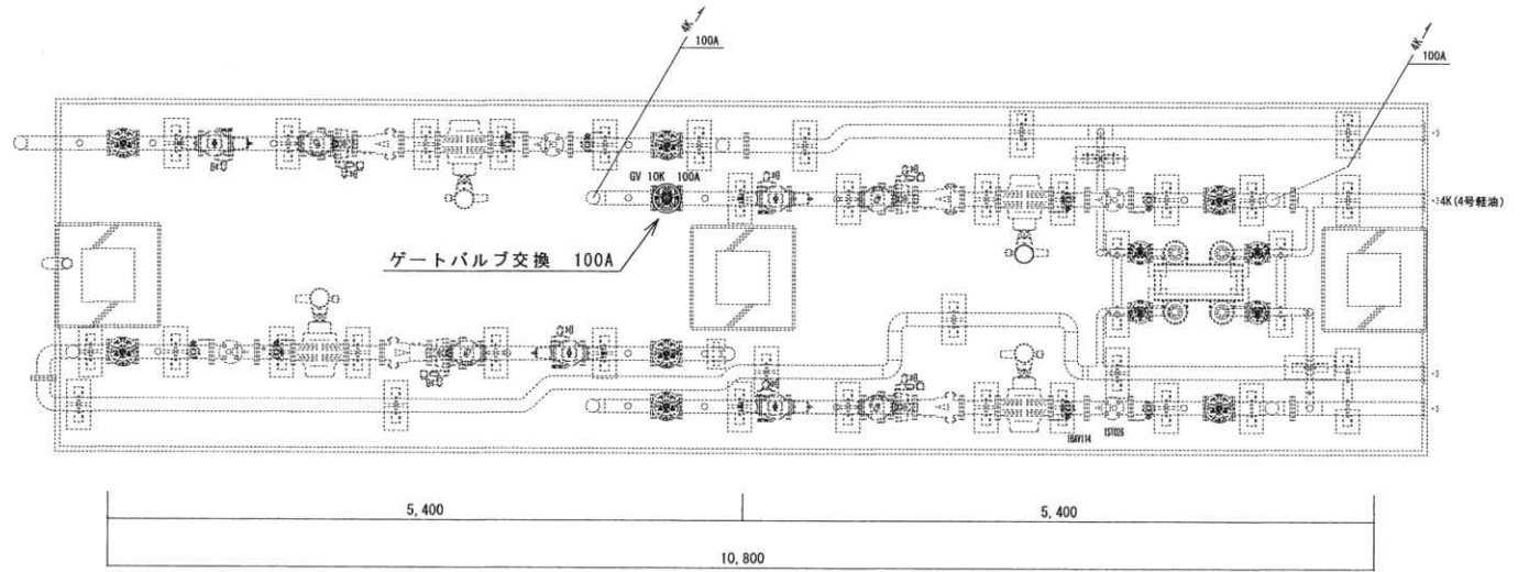
アイランド3 平面図 S=1:50
