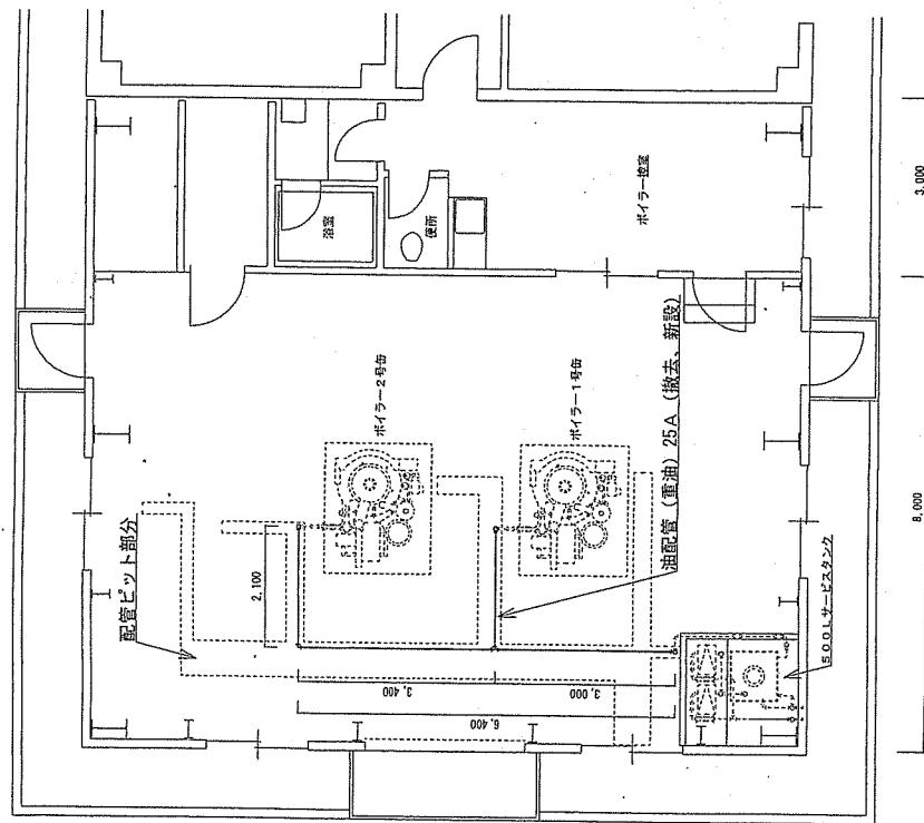
ボイラー室平面図 S=1/100
