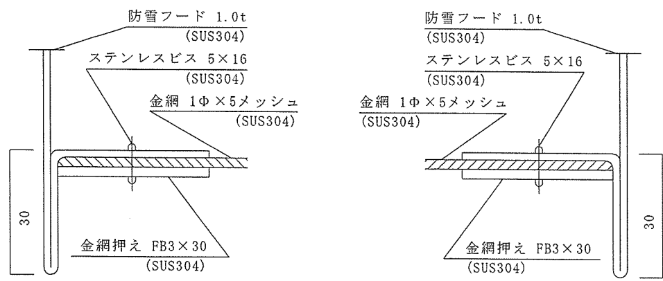
B 詳細図
