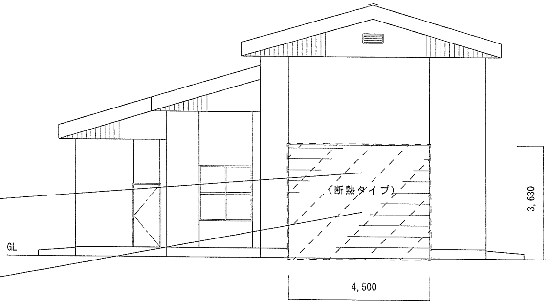
北側立面図
