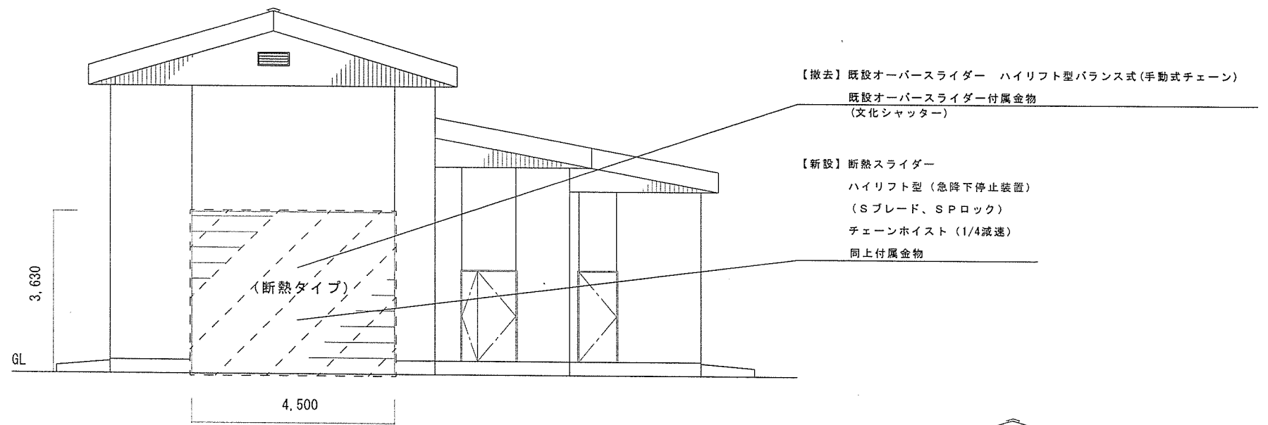
南側立面図
