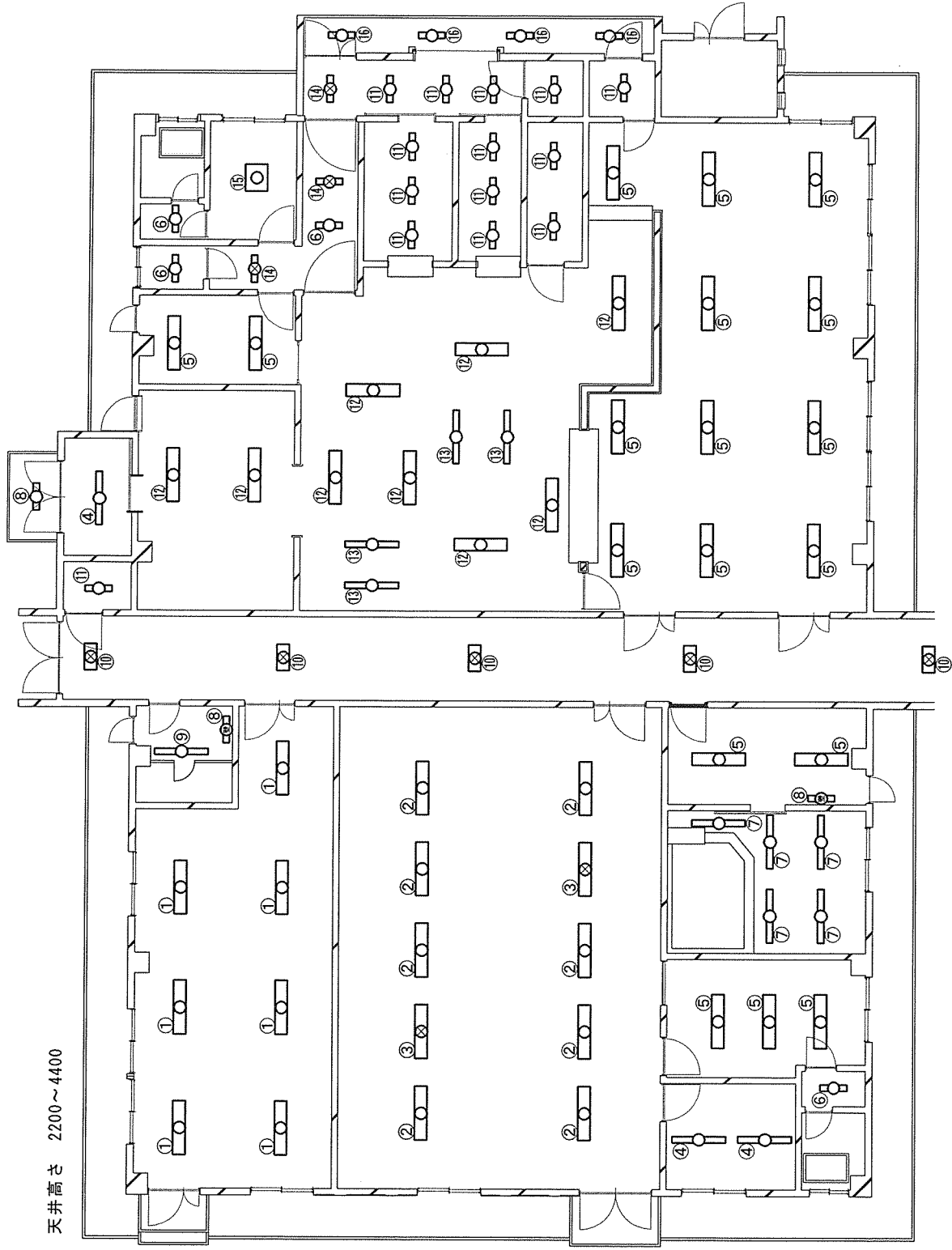
#4管理棟平面図・取付図
