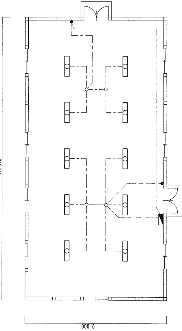
#84保管庫平面図 S=1:100
