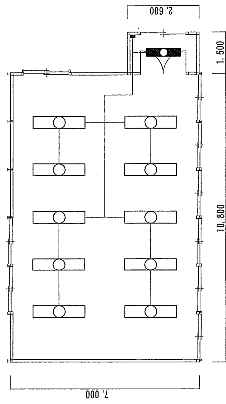
#61外来宿舍平面図 S=1:100
