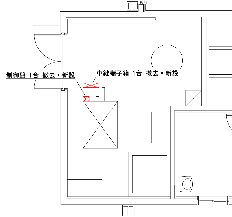
機械室詳細図 1/500
