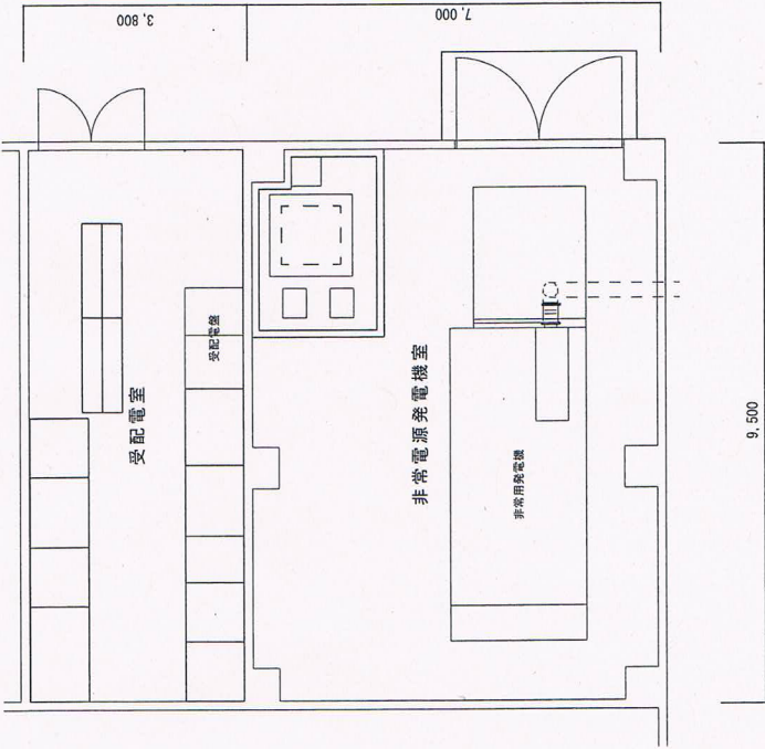
自家発電機室平面図 S=1/100
