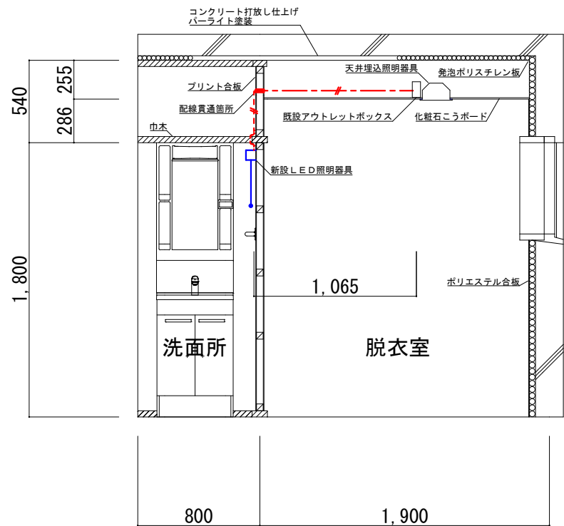
A-B断面図 1/50
