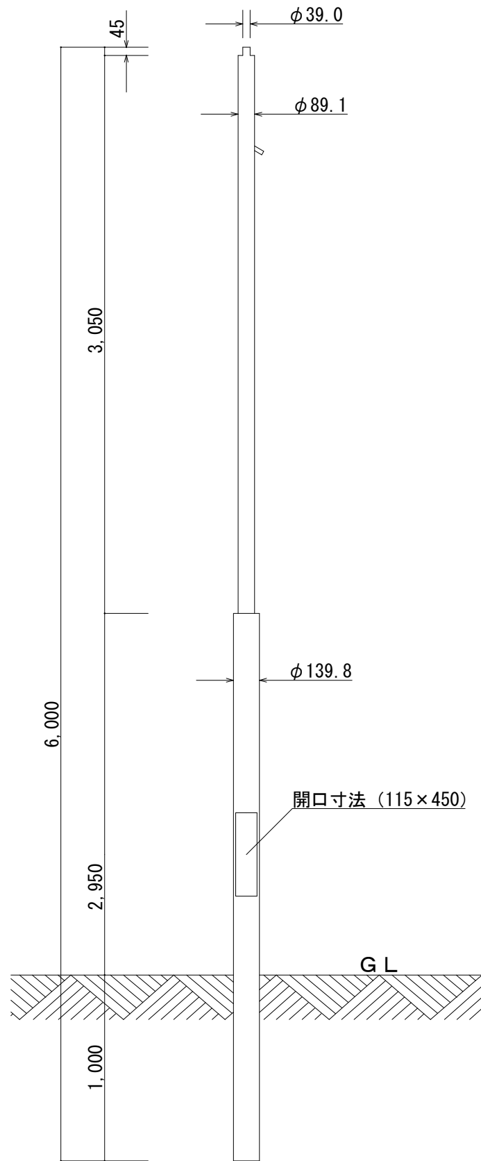
既設ポール立面図 1/50
