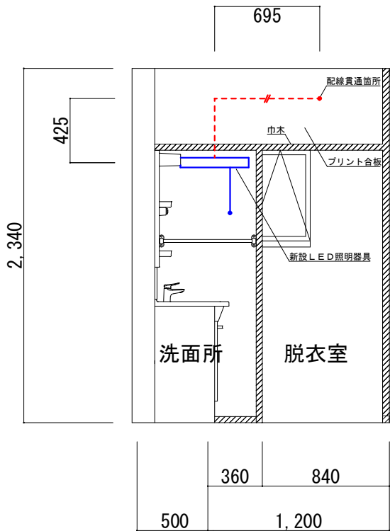
C-D断面図 1/50
