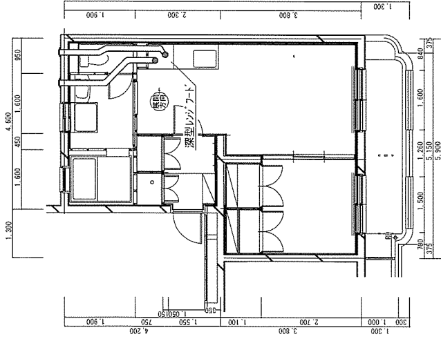
B棟(aタイプ)平面図 S=1:100
