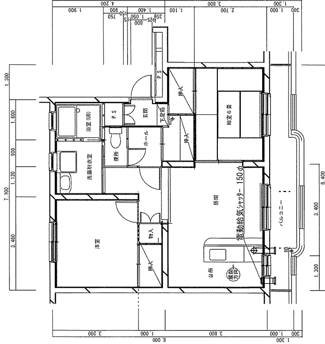
B棟(bタイプ)平面図 S=1:100
