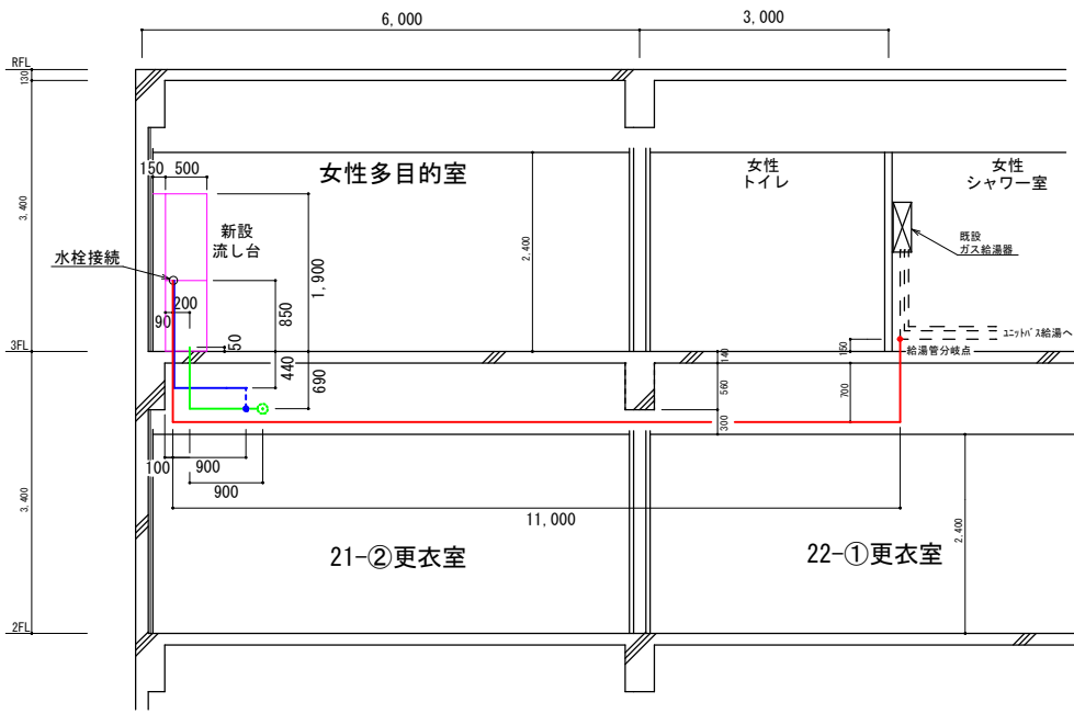
配管断面図
