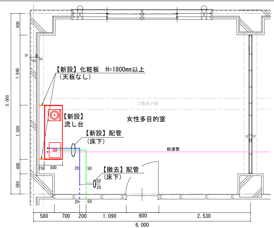
女性多目的室改修図
