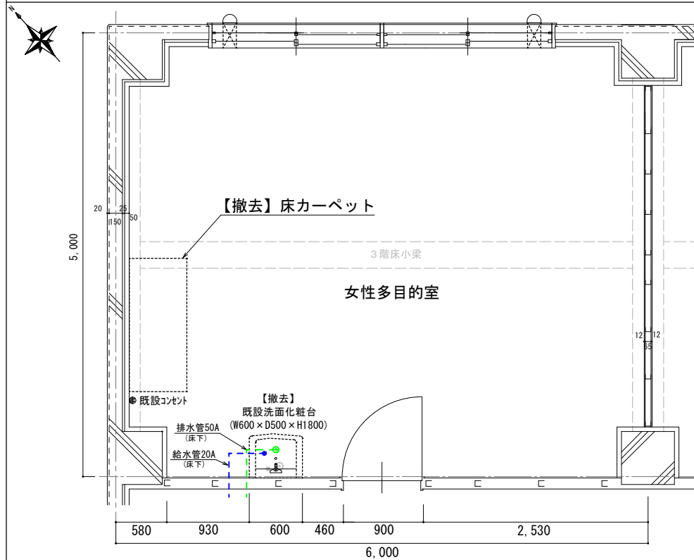
女性多目的室現況図
