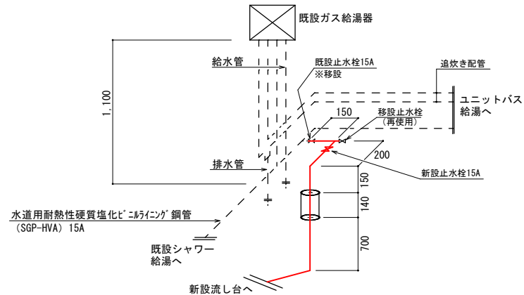
給湯配管図
