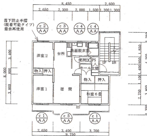
cタイプ平面図 (標準図) S=1:200
