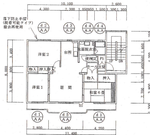
dタイプ平面図 (標準図) S=1:200
