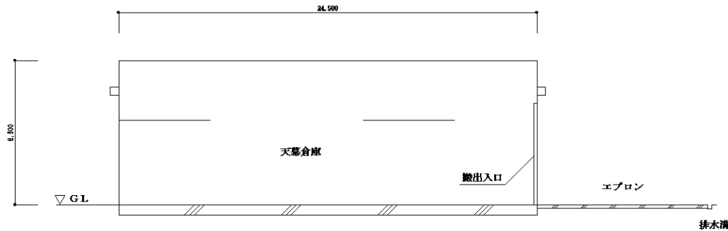
天幕倉庫断面図 S=1/200
