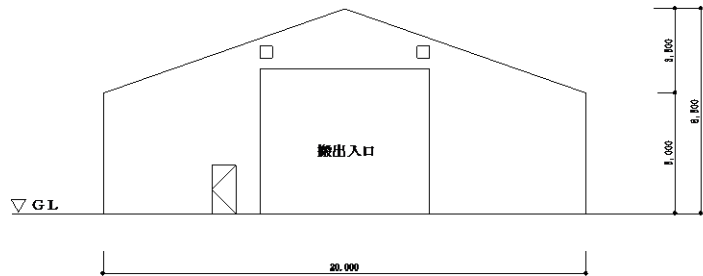
天幕倉庫搬入口側立面図 S=1/200
