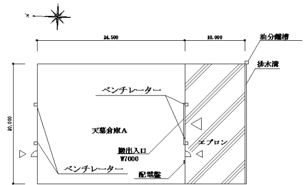
天幕倉庫A平面図 S=1/400
