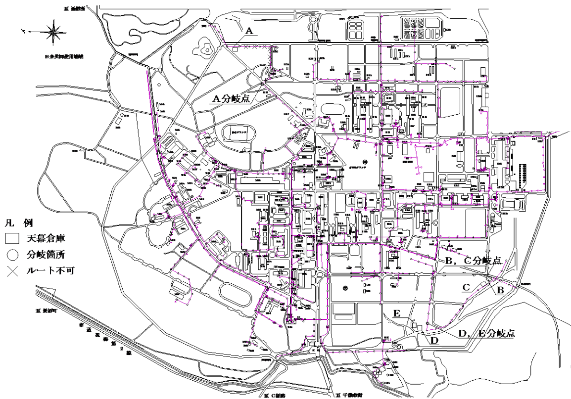
電気系統図 S=1/12000
