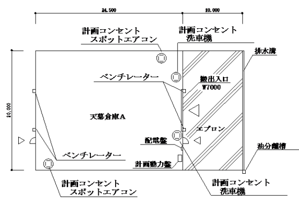
天幕倉庫 平面図 S=1/400
