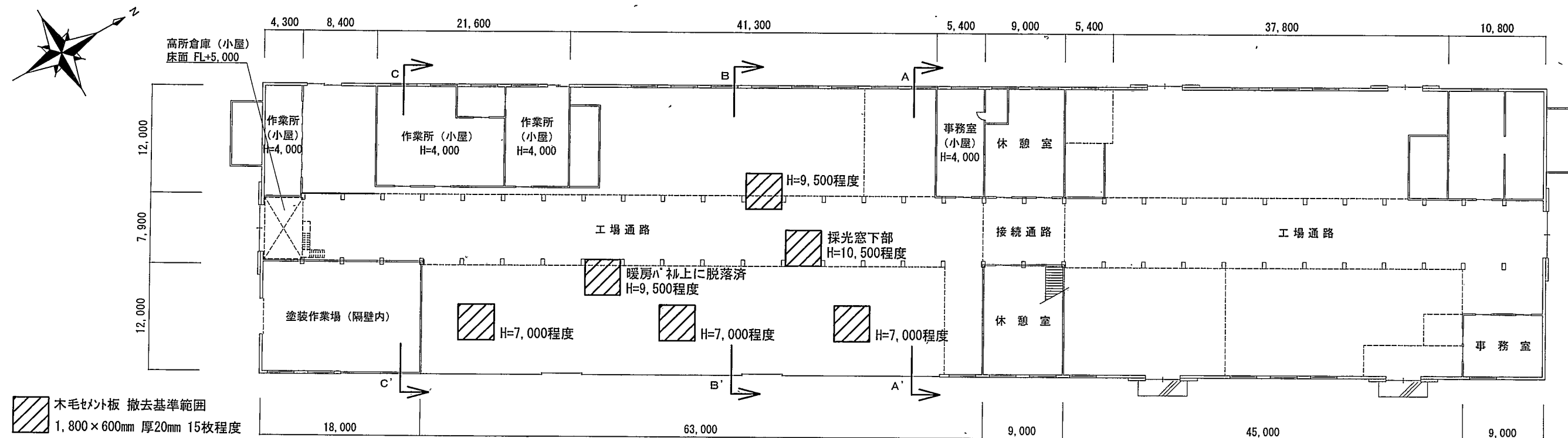
# 3 5 工場 防護ネット設置基準高さ S=1:500
