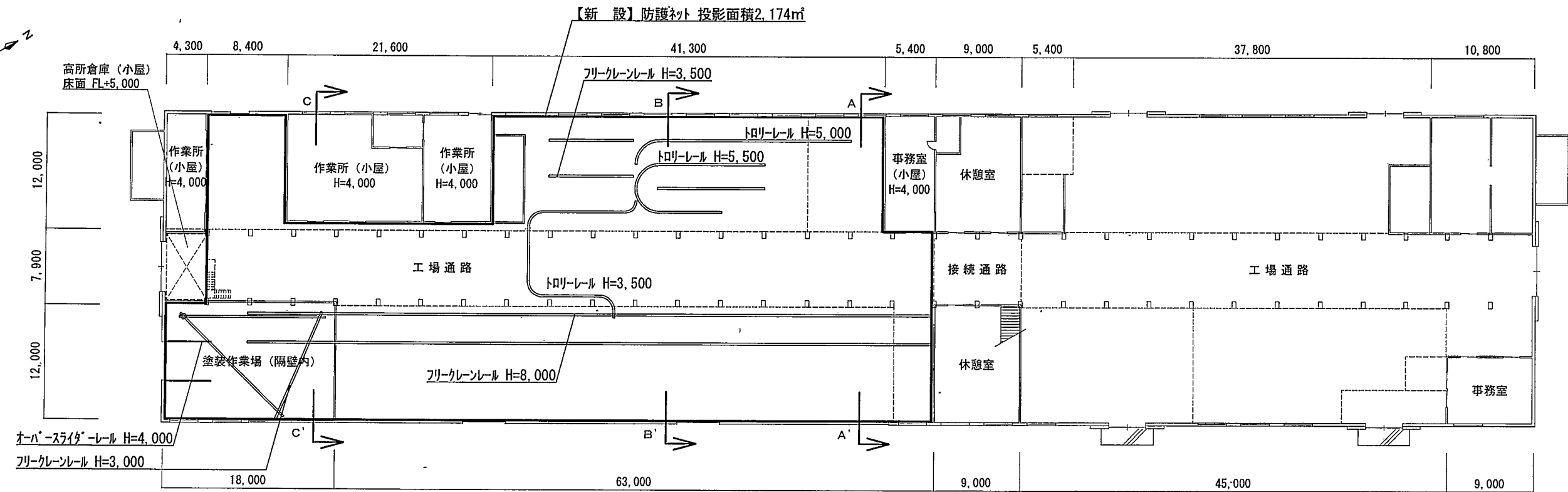
#35工場 機械器具設備図 S=1:500
