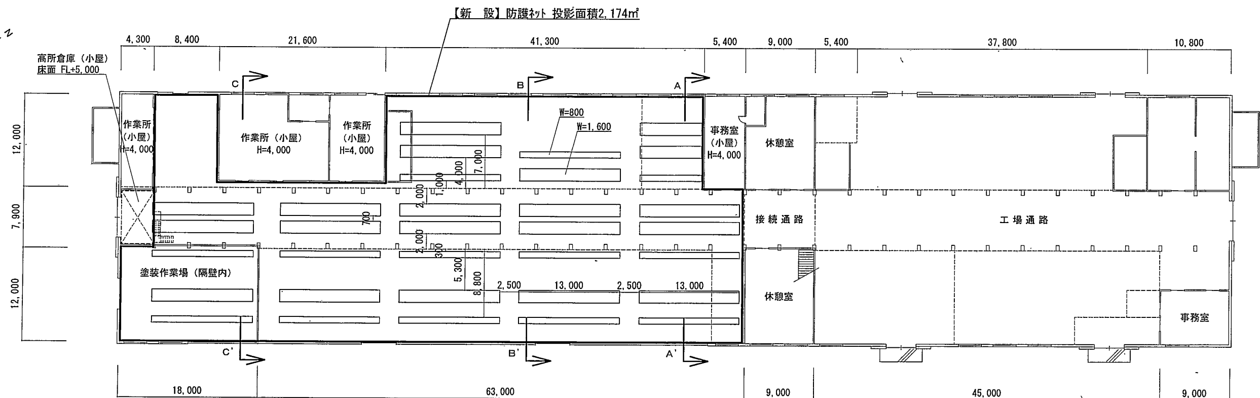
#35工場 暖房パネル配置図 S=1:500
