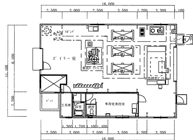
既設 第2ボイラー室 S=1:200
