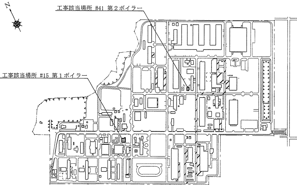
島松駐屯地配置図 S=1:8000
