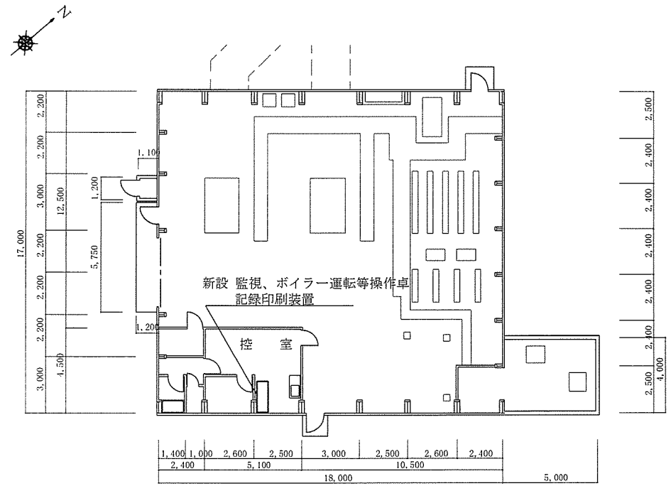
既設 第1ボイラー室 S=1:200
