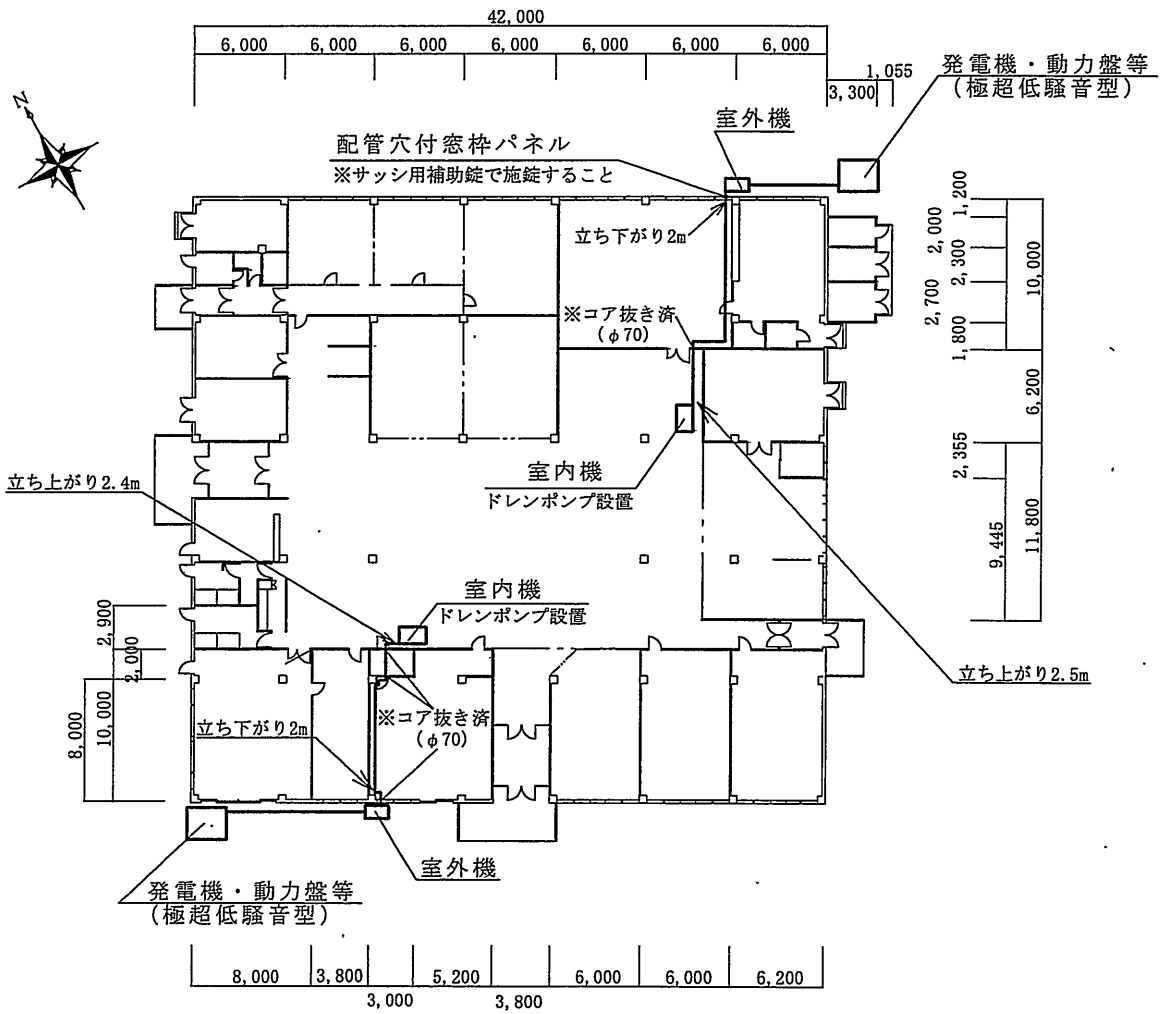
厚生施設平面図 S=1:500
