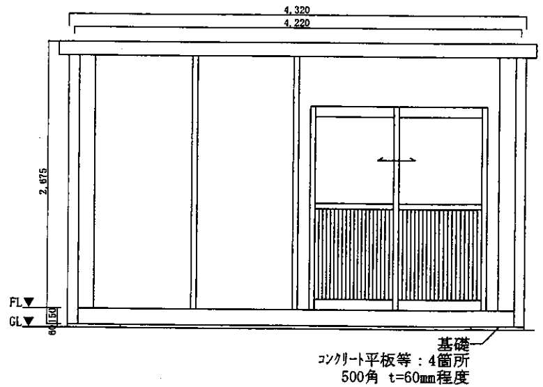
立面図 S=1:50
