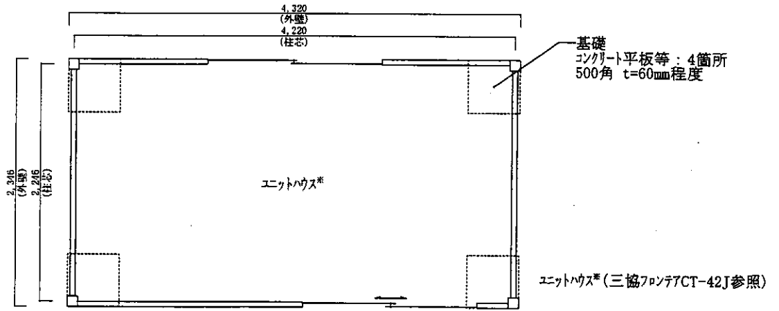
平面図 S=1:50
