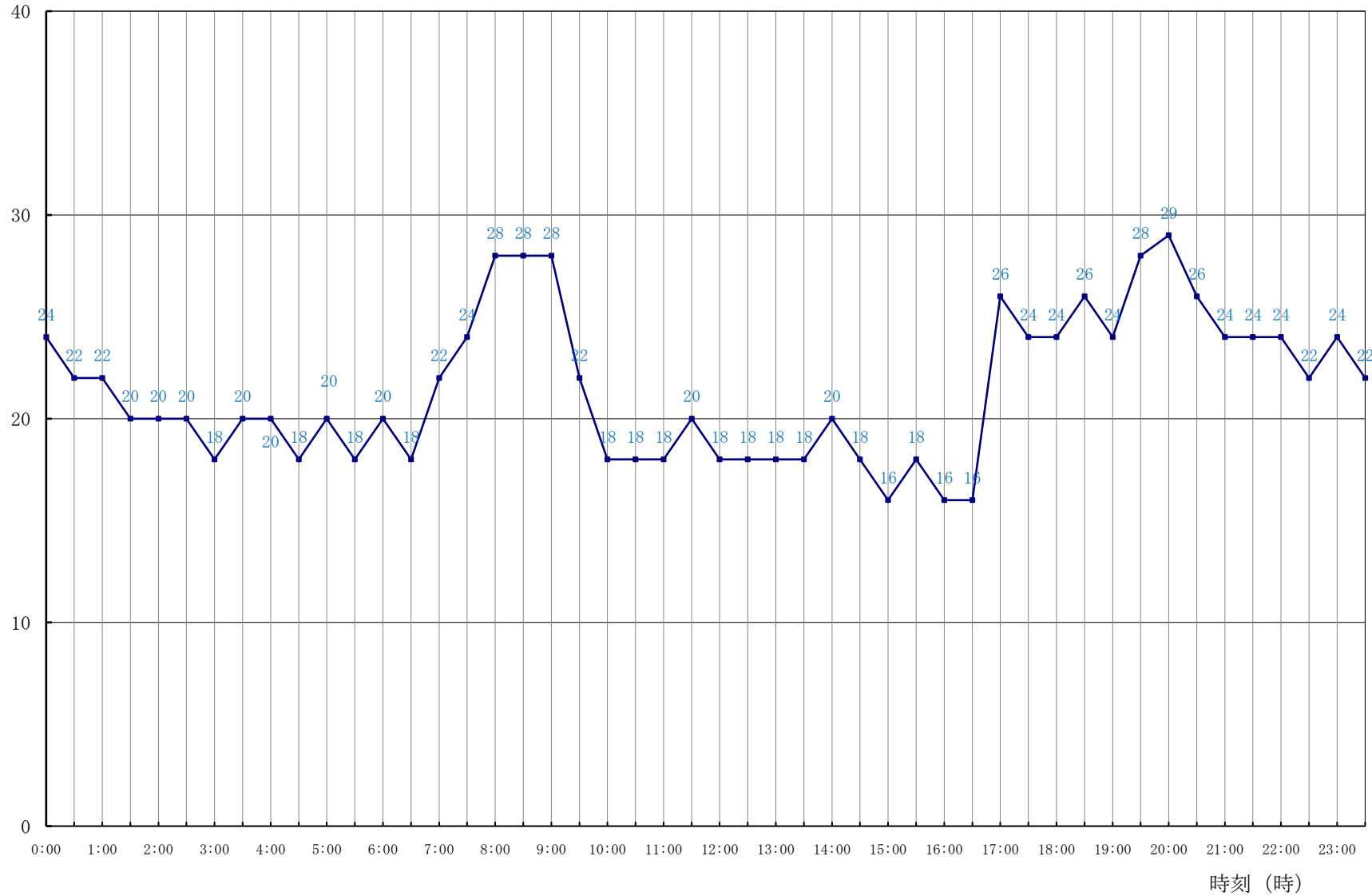
令和6年12月～令和7年11月最大負荷日のロードカーブ (最大電力29kW)
