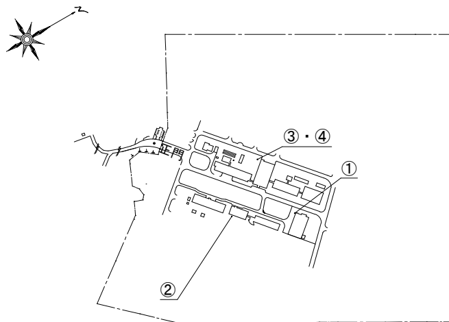
配置図 S=1/10,000
